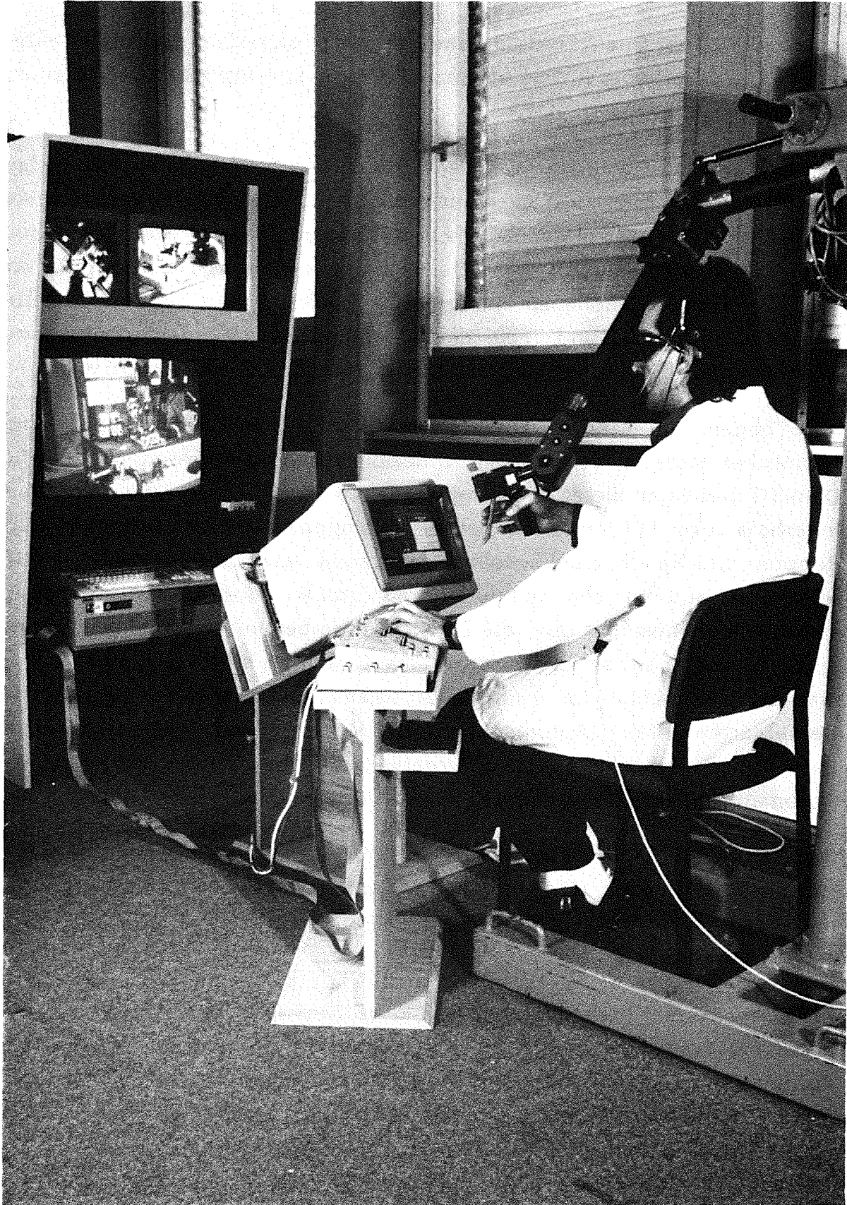
Bild 4: Mensch/Maschine-Schnittstelle des Telemanipulatorsystems DISTEL
