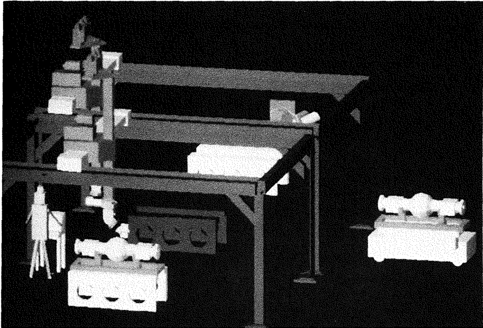
Bild 12: Simulationsbild ROBCAD
