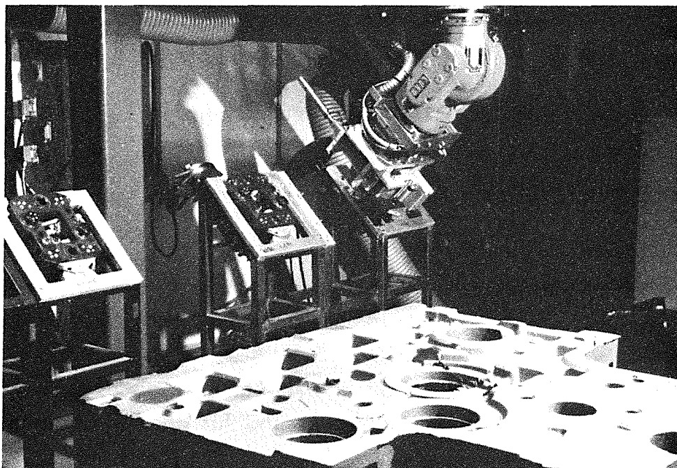
Bild 9: COMETOS mit einer Druckmaschinenseitenwand
