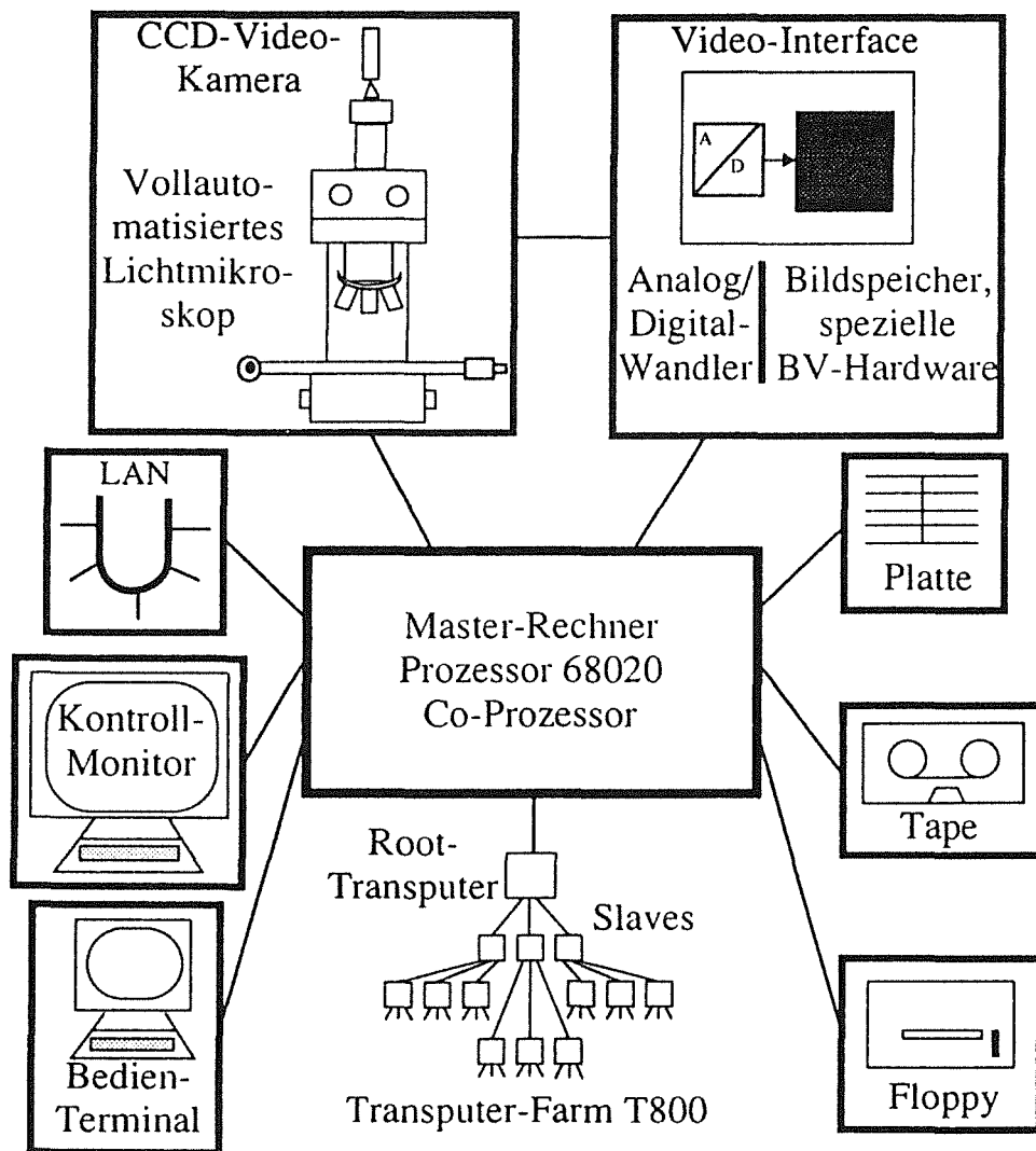
Bild 3: Übersichtsskizze des Strukturvermessungssystems
